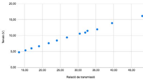
Evolució de la tensió elèctrica en funció de la Rel. Transmissió
