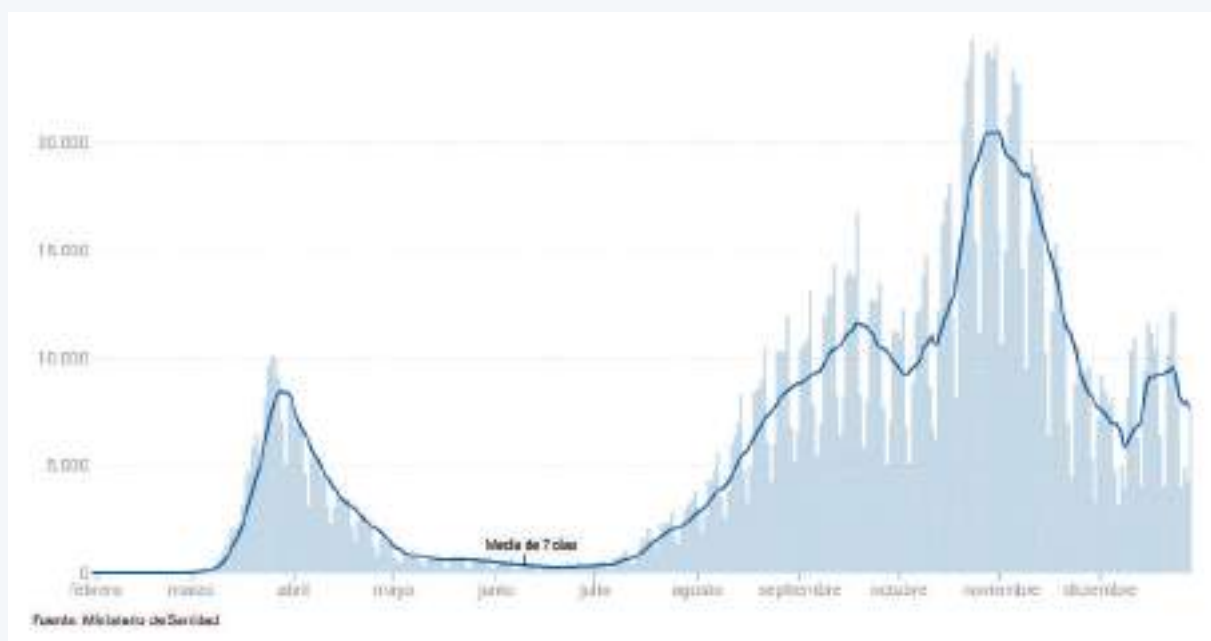
Evolució de contagis a Espanya en 2020 (eldiario.es)
