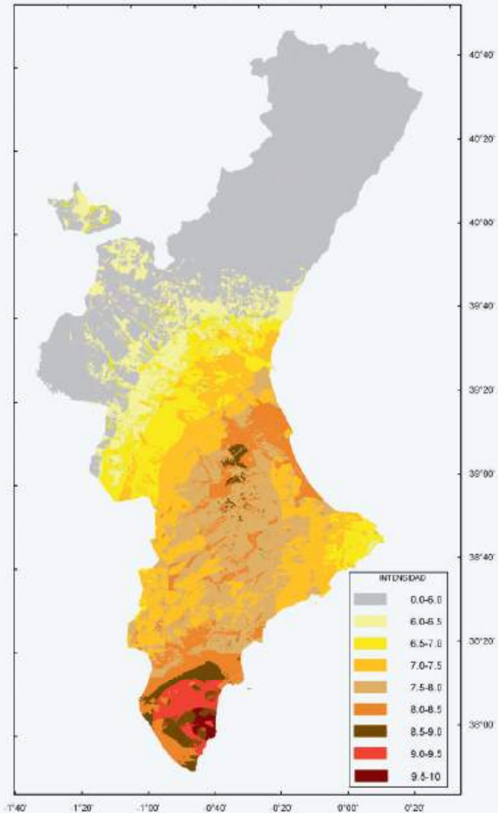
Mapa d'intensitat sísmica esperada en la Comunitat Valenciana per a un període de retorn de 500 anys (elaborat per Juan José Giner Caturla, Universitat d'Alacant)
