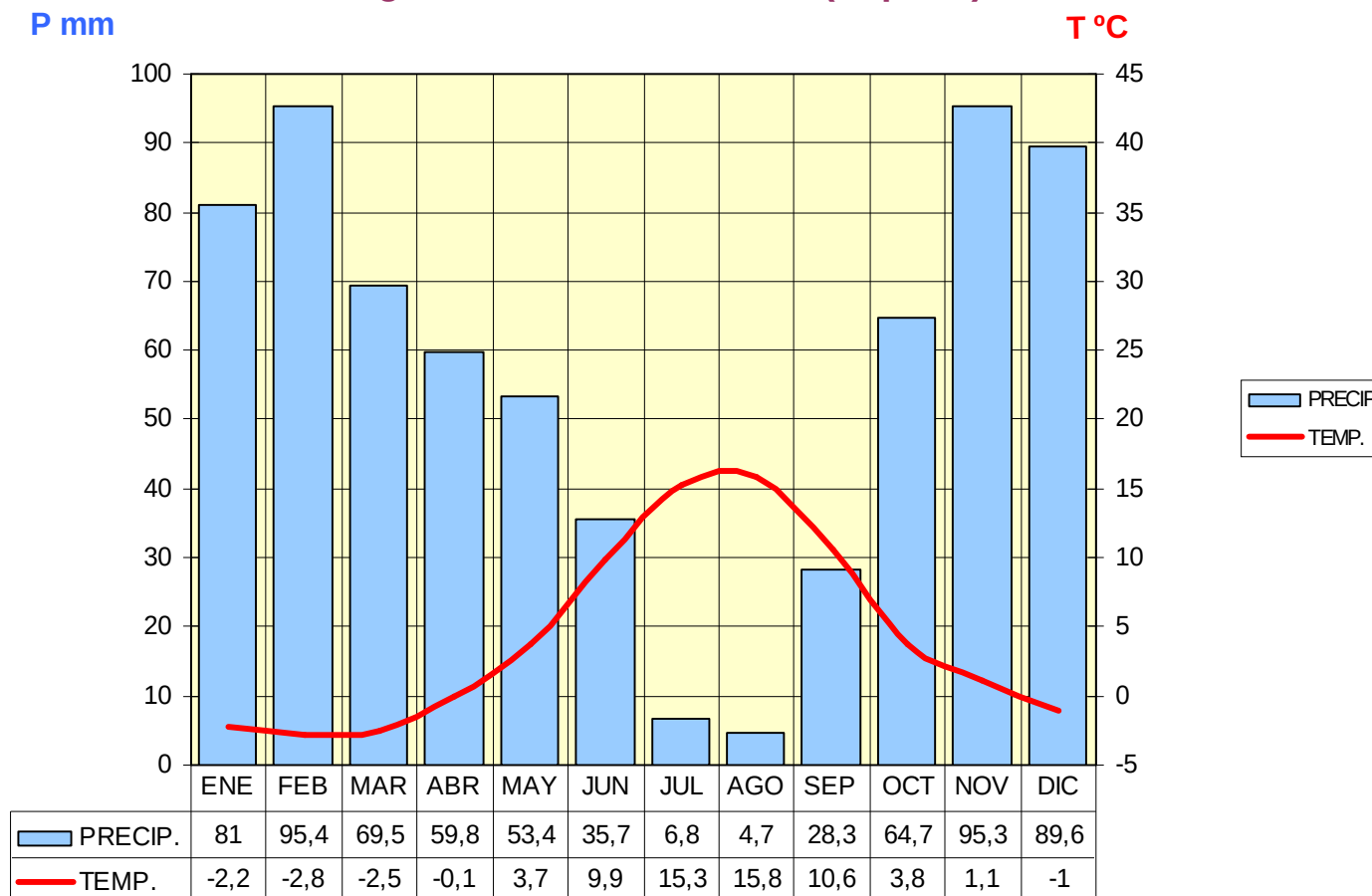
Climograma de Sierra Nevada (España)
