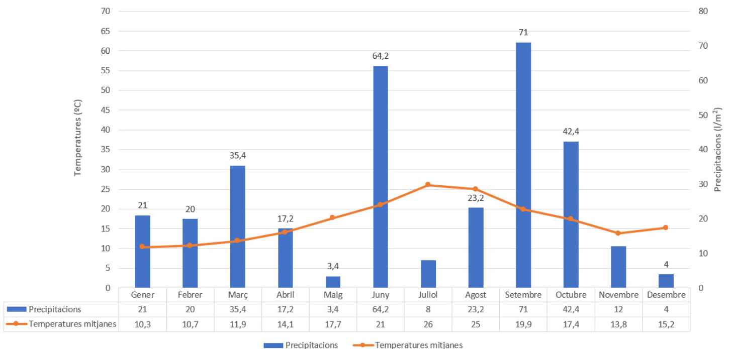
Diagrama ombrotèrmic d'Ibi (IES la Foia) en 2024
