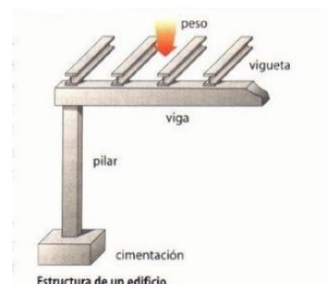
Estructura de un edificio.
