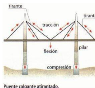
Puente colgante atirantado.
