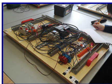
Panells elèctrics per a fer pràctiques
