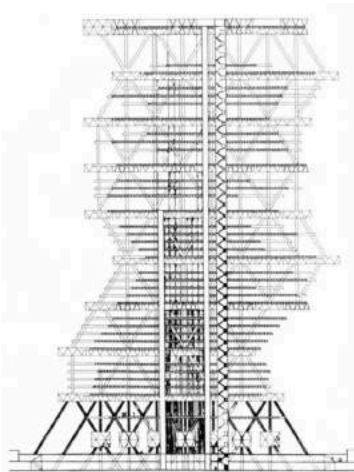
La Torre de la Ciudad, diseñada por Louis Kahn con la arquitecta Anne Tyng en Filadelfia (1952-1957) y nunca realizada, es un rascacielos geodésico, estabilizado por suelos de hormigón tetraédricos.
