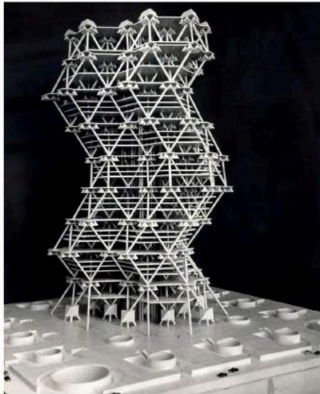
La Torre de la Ciudad, diseñada por Louis Kahn con la arquitecta Anne Tyng en Filadelfia (1952-1957) y nunca realizada, es un rascacielos geodésico, estabilizado por suelos de hormigón tetraédricos.
